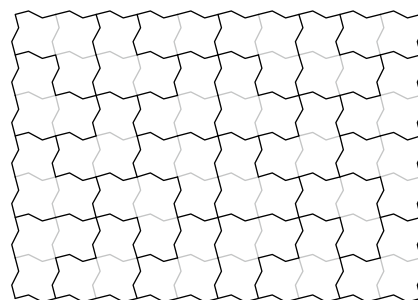
Ankerverbund, maschinelle Verlegung Die Liefereinheit (Stärken 8 cm und 10 cm) entspricht ca. 0,91 m 2 (115 cm x 81 cm).
