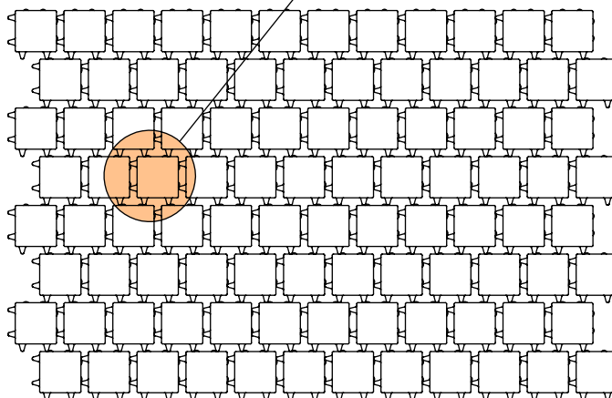
Ökodur-Rasenfuge, maschinelle Verlegung im Läuferverband mit 30 mm Fuge
