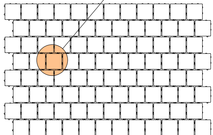
Ökodur-Drainfuge, maschinelle Verlegung im Läuferverband mit 10 mm Fuge
